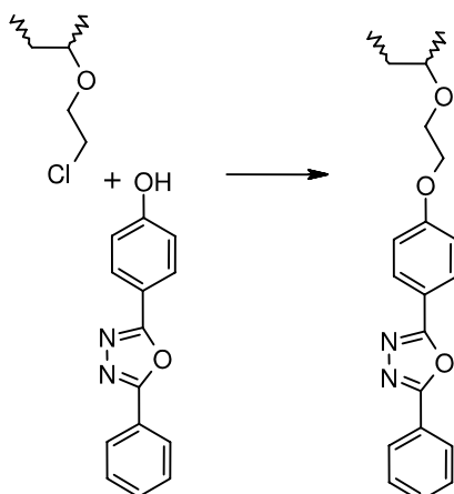
الشكل (6-1): تغيير زمر الكلور المتدلية مع 2-(4-هيدروكسي
